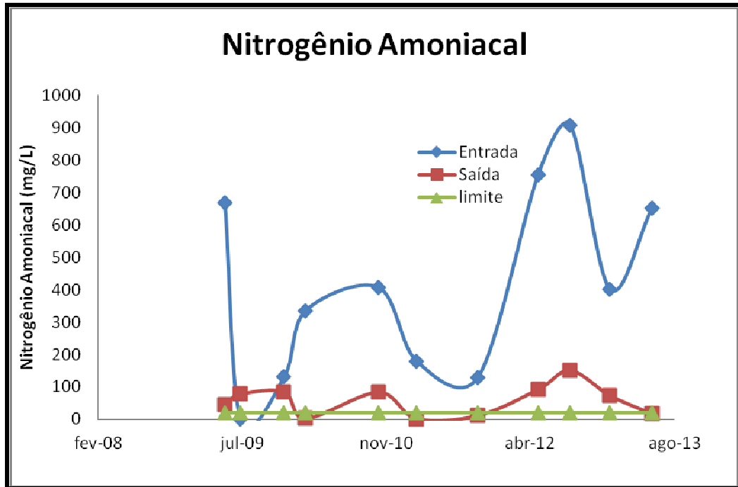
Figura 18: Nitrogênio Amoniacal entrada e saída ETE.
