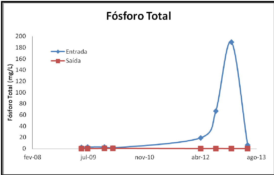
Figura 16: Fósforo Total entrada e saída ETE.
