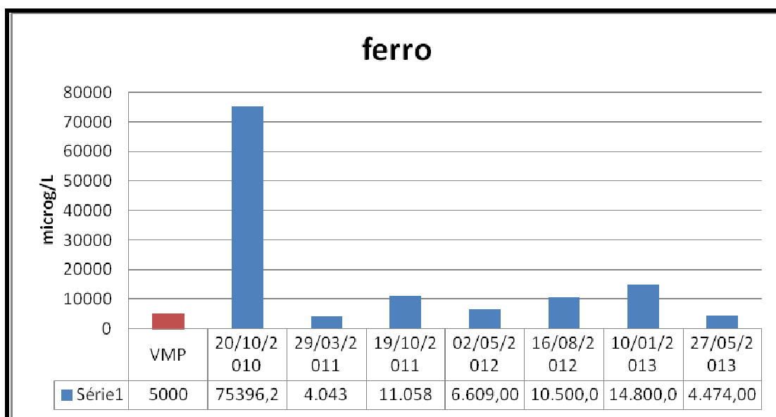
Figura 21: Ferro PZM 03.
