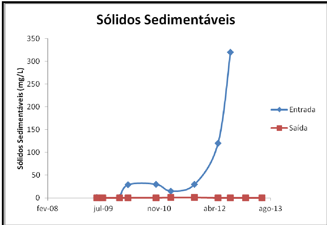
Figura 12: Sólidos Sedimentáveis entrada e saída ETE.
