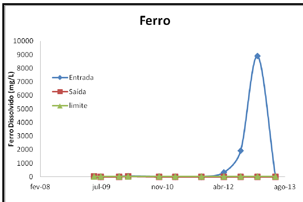
Figura 15: Ferro entrada e saída ETE.
