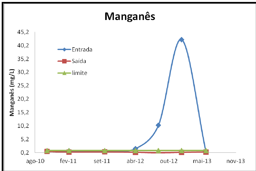
Figura 17: Manganês entrada e saída ETE.
