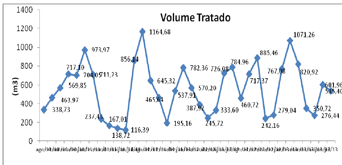
Figura 06: Vazão de chorume tratado na ETE do Cirsures, até julho de 2013.
