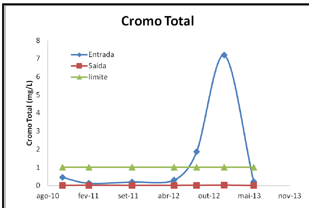
Figura 14: Cromo Trivalente entrada e saída ETE.
