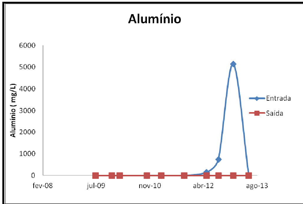
Figura 08: Alumínio entrada e saída ETE.
