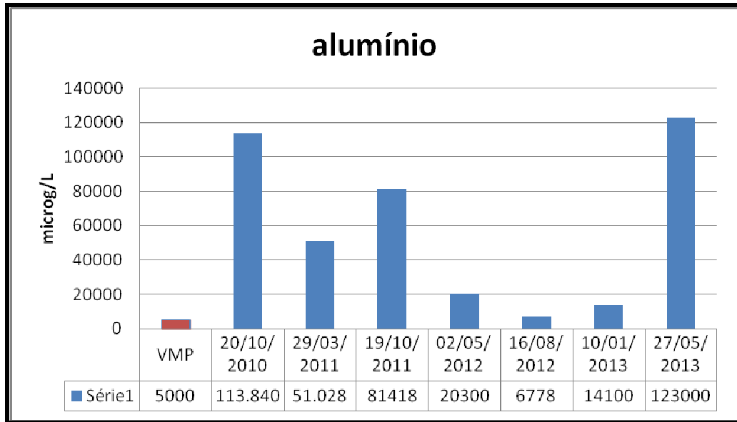
Figura 20: Alumínio PZM 02.
