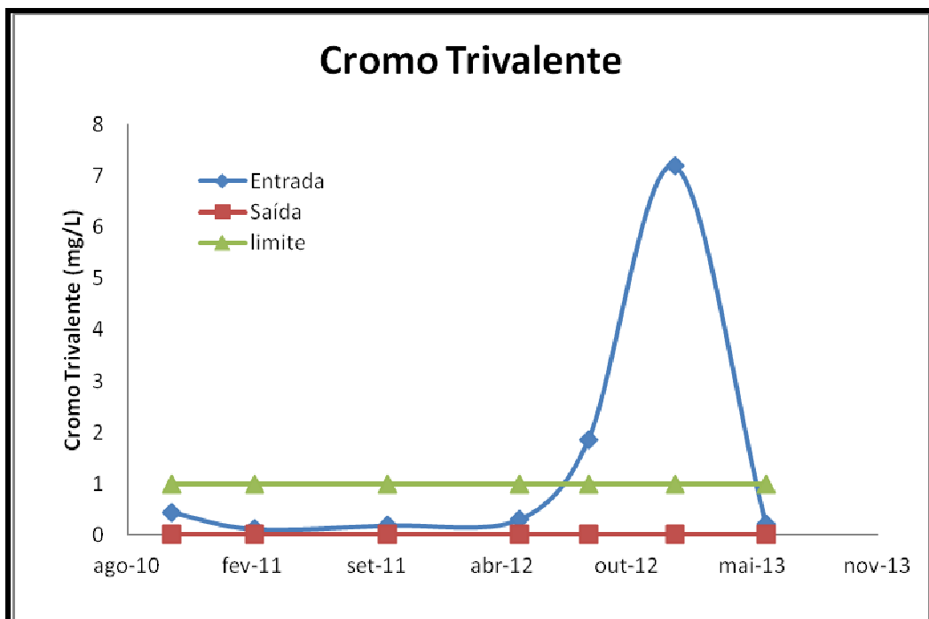
Figura 13: Cromo Trivalente entrada e saída ETE.
