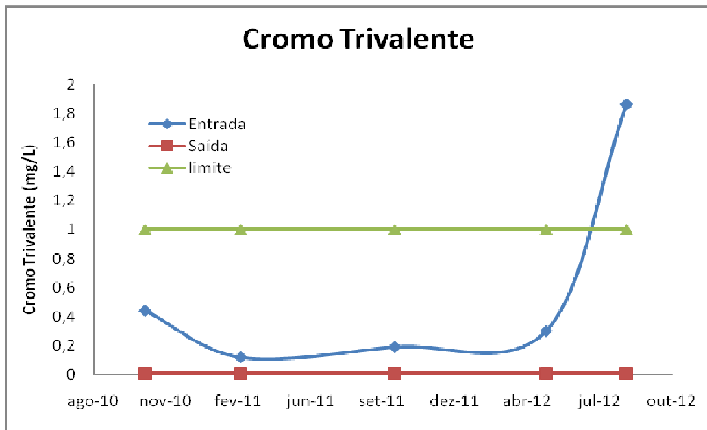
Figura 14: Cromo Trivalente entrada e saída ETE.
