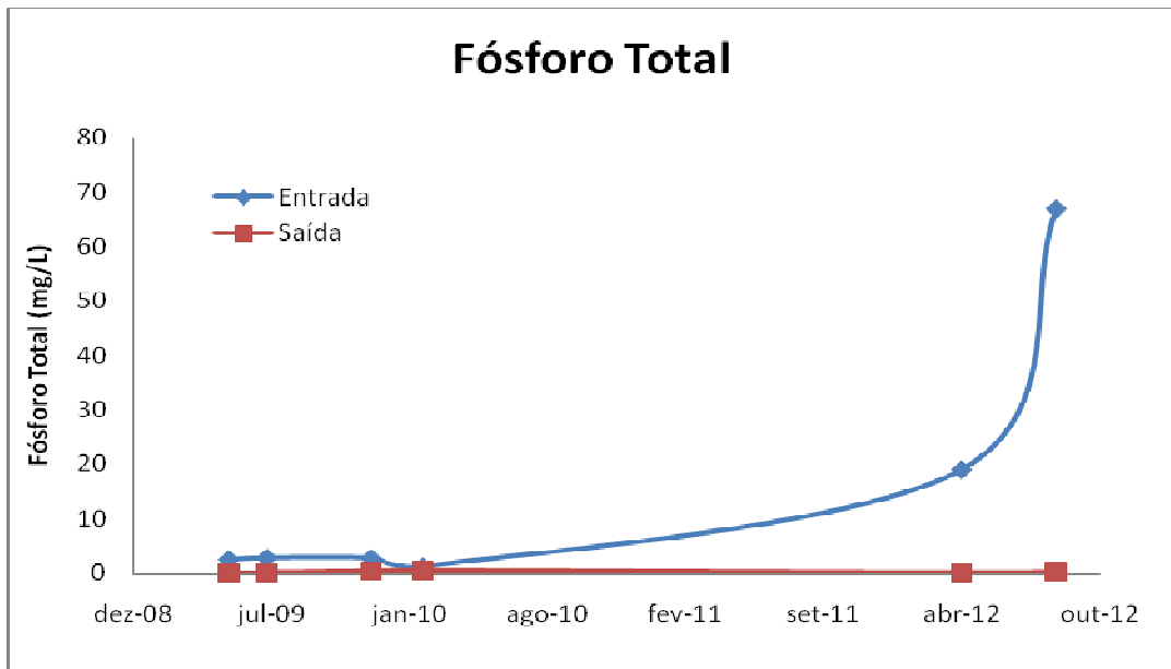
Figura 17: Fósforo Total entrada e saída ETE.
