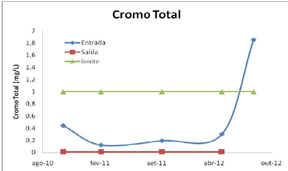
Figura 15: Cromo Trivalente entrada e saída ETE.
