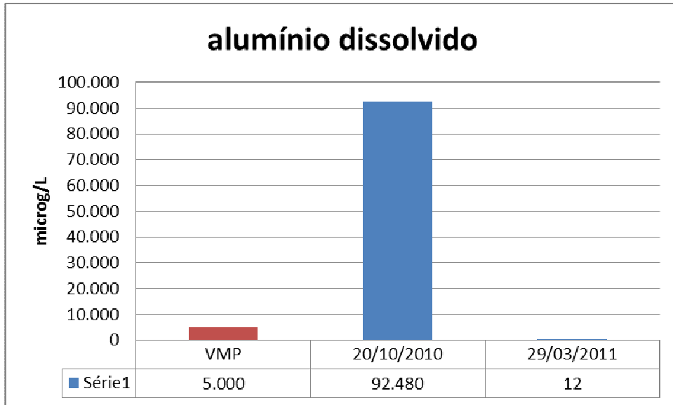
Figura 22: Alumínio Dissolvido PZ 01.
