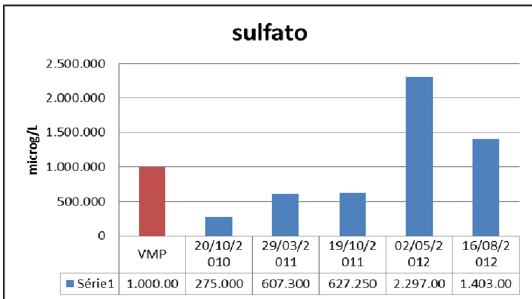
Figura 32: Sulfato PZM 02.
