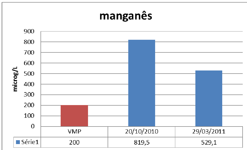
Figura 25: Manganês PZ 01.
