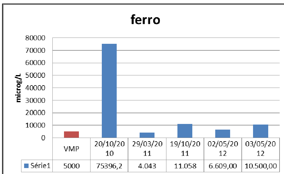
Figura 33: Ferro PZM 03.
