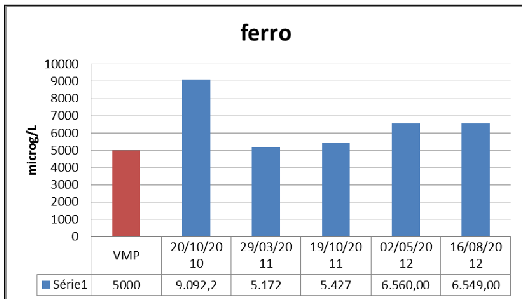
Figura 30: Ferro PZM 02.
