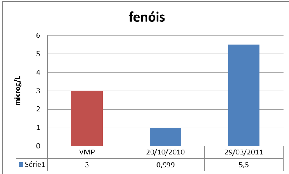
Figura 28: Fenóis PZ 01.
