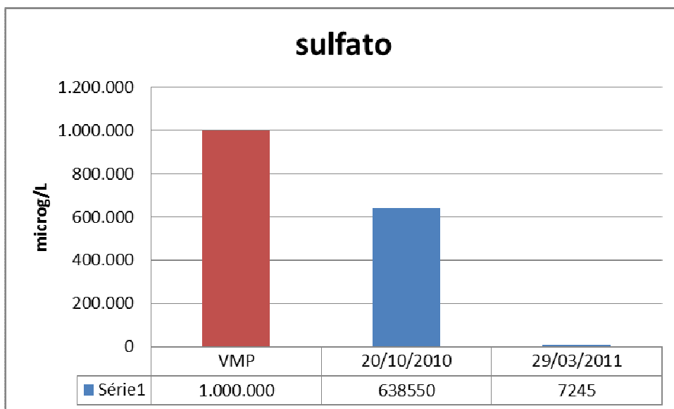
Figura 27: Sulfato PZ 01.
