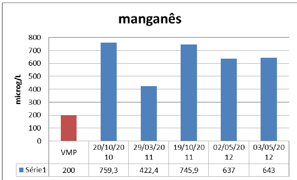
Figura 34: Manganês PZM 03.
