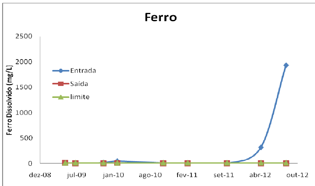
Figura 16: Ferro entrada e saída ETE.
