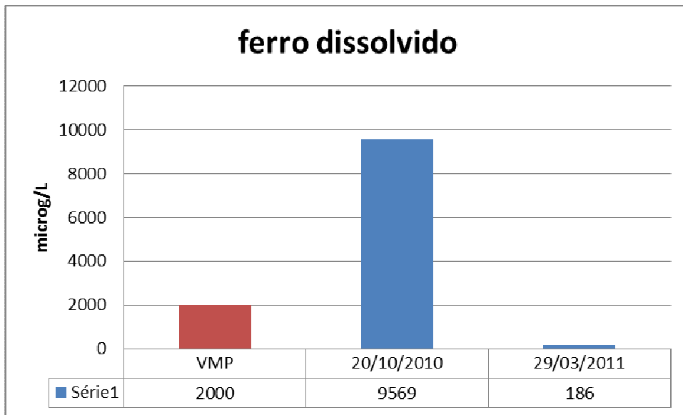
Figura 24: Ferro Dissolvido PZ 01.
