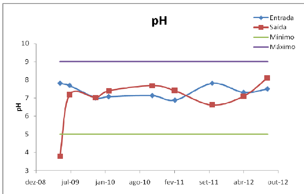
Figura 10: pH entrada e saída ETE.
