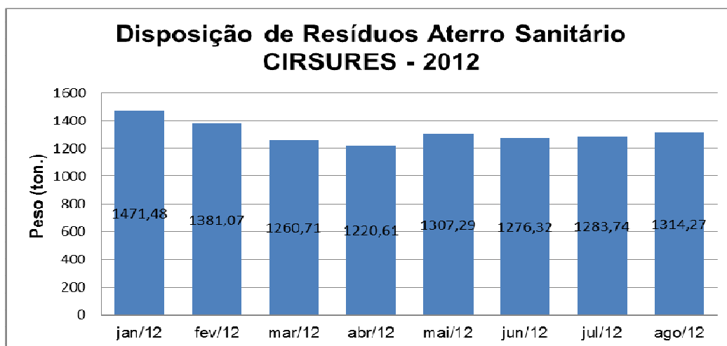
Figura 37: Gráfico de disposição de resíduos no aterro sanitário do Cirsures.
