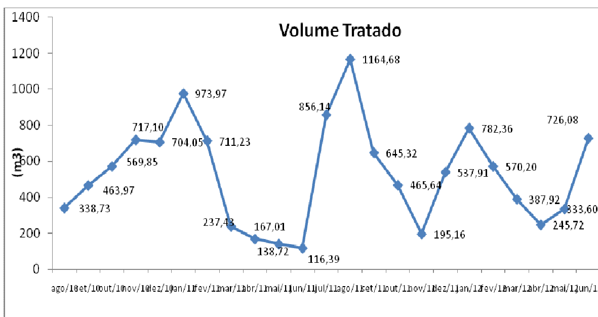
Figura 7- Vazão de chorume tratado na ETE do Cirsures.
