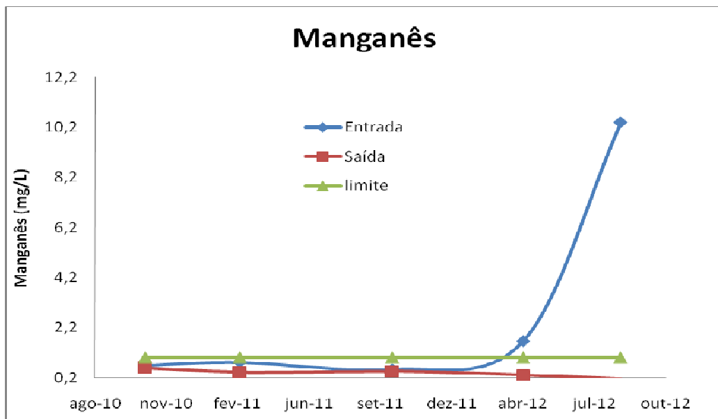
Figura 18: Manganês entrada e saída ETE.
