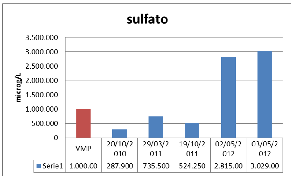
Figura 35: Sulfato PZM 03.
