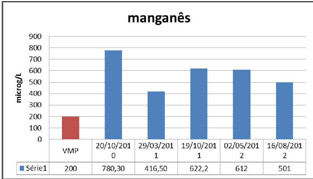
Figura 31: Manganês PZM 02.
