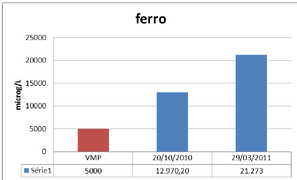
Figura 23: Ferro PZ 01.
