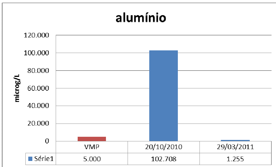
Figura 21: Alumínio PZ 01.
