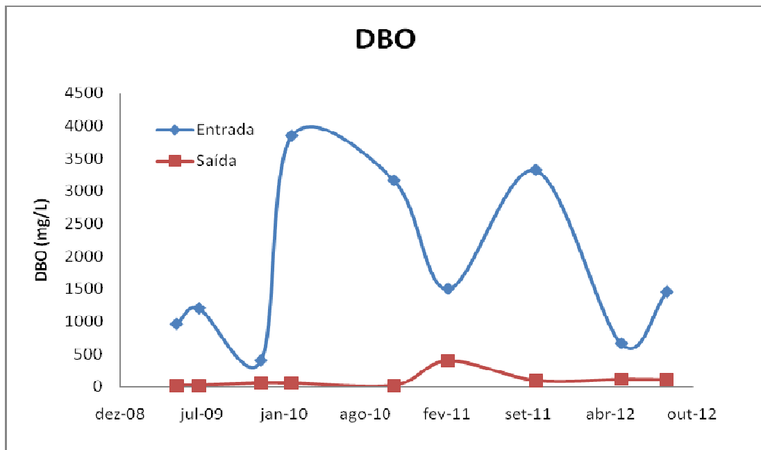
Figura 12: DBO entrada e saída ETE.
