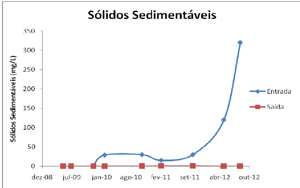
Figura 13: Sólidos Sedimentáveis entrada e saída ETE.
