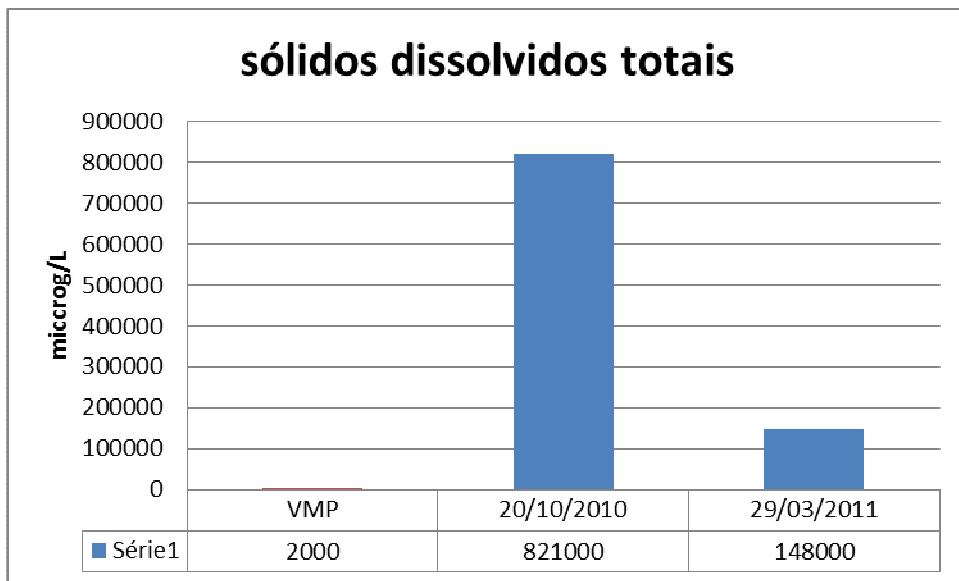
Figura 29: Sólidos Dissolvidos Totais PZ 01.
