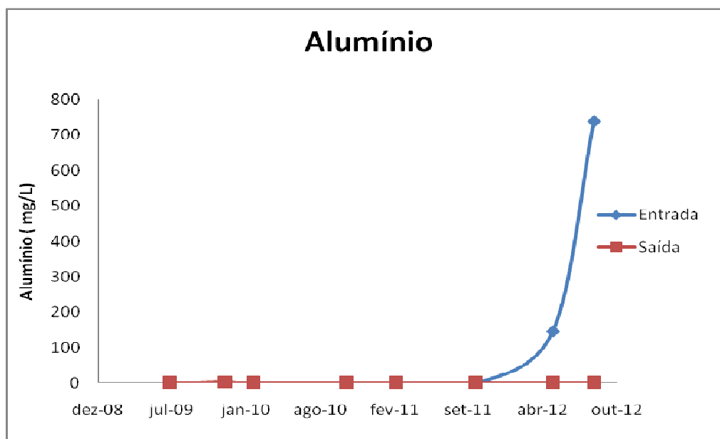
Figura 09: Alumínio entrada e saída ETE.
