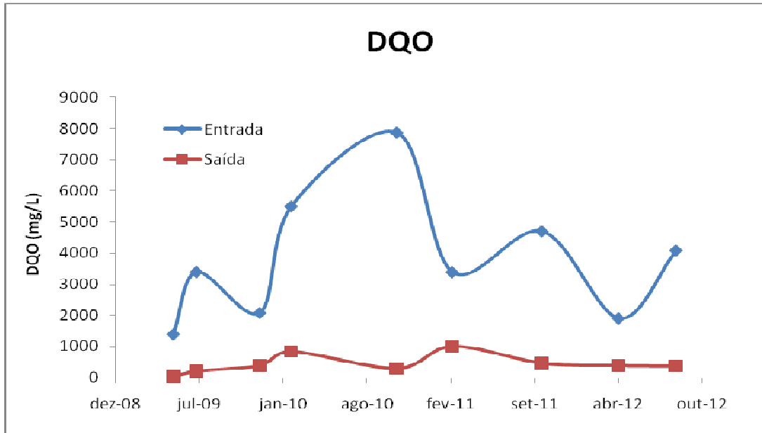
Figura 11: DQO entrada e saída ETE.
