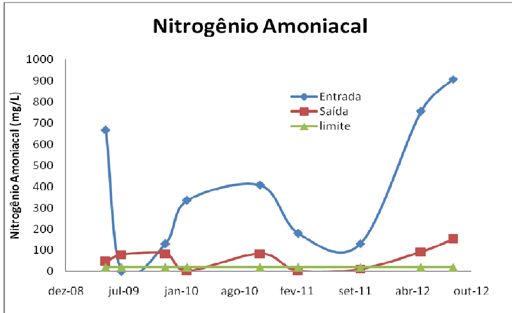
Figura 19: Nitrogênio Amoniacal entrada e saída ETE.
